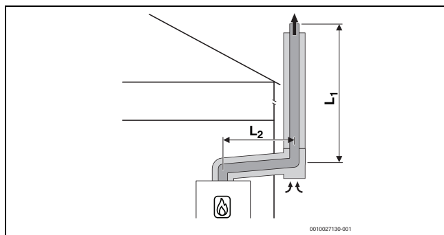
Мал. 13 Система транспортування повітря для горіння та відпрацьованих газів у концентричних трубах відповідно до C_{53x} на зовнішній стіні
