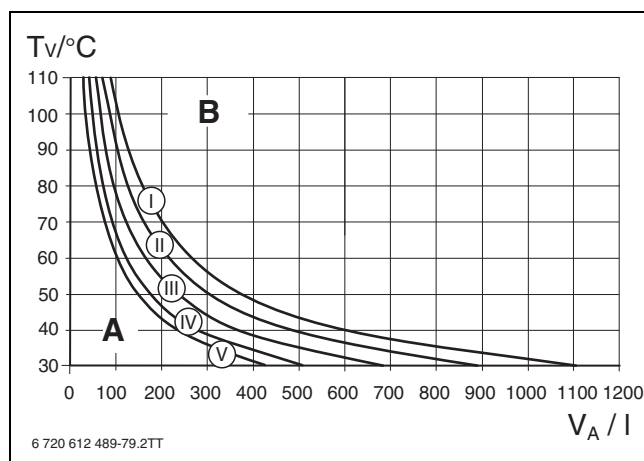
Мал. 25 Характеристична крива мембранного компенсаційного бака
