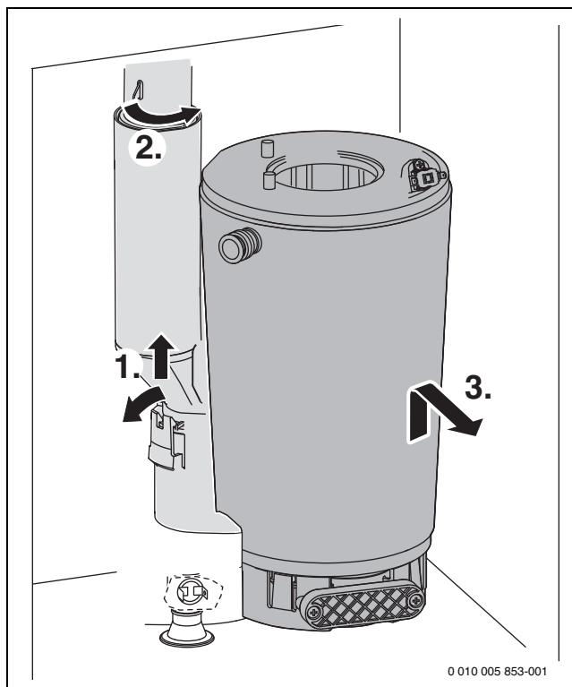
Мал. 84 Демонтаж котлового блока, який включає камеру згоряння і теплообмінник
