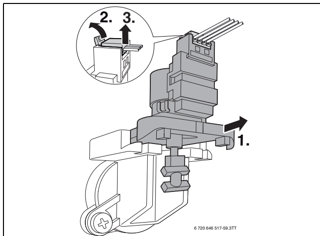
Мал. 73 Зняття мотора 3-ходового клапана
