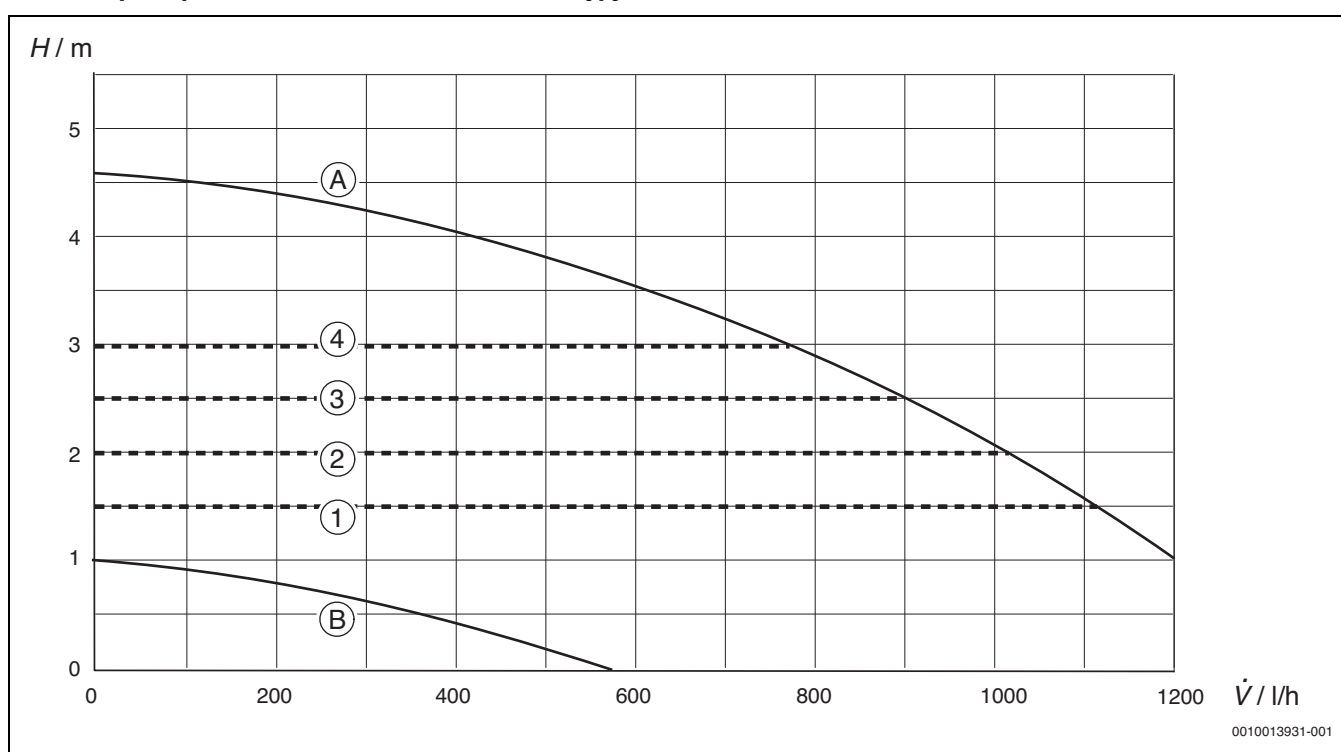
Мал. 89 Характеристики насоса та криві характеристик насоса
