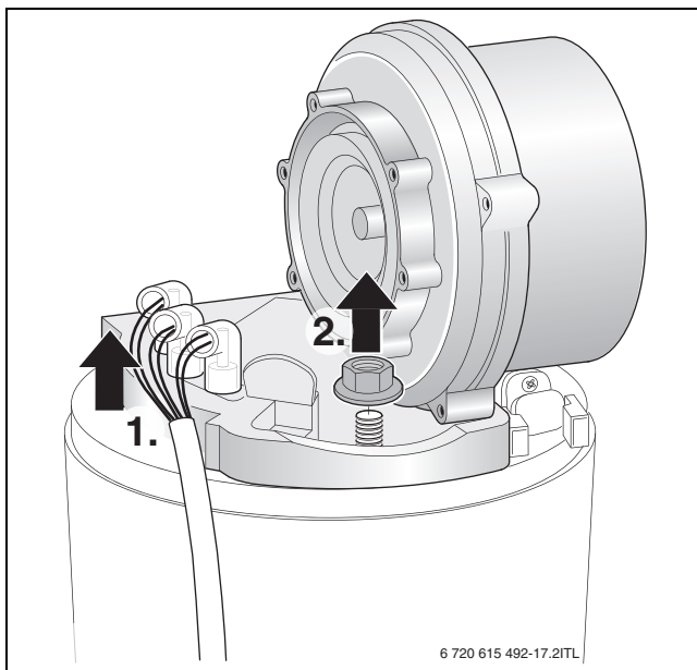
Мал. 60 Виймання вентилятора
