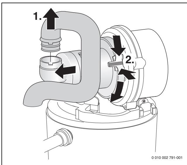
Мал. 59 Демонтаж впускної труби та змішувальної камери
