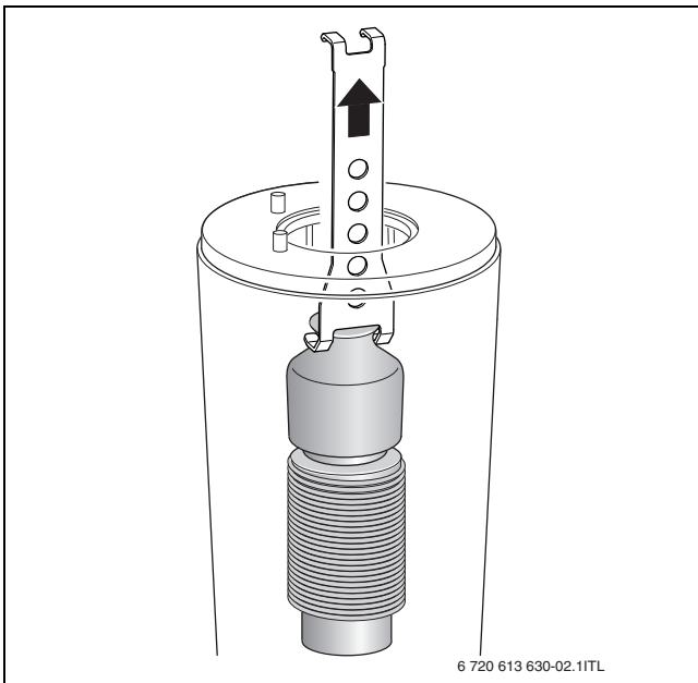
Мал. 62 Виймання верхнього елемента теплообмінника, що служить для оптимізації розподілювання тепла
