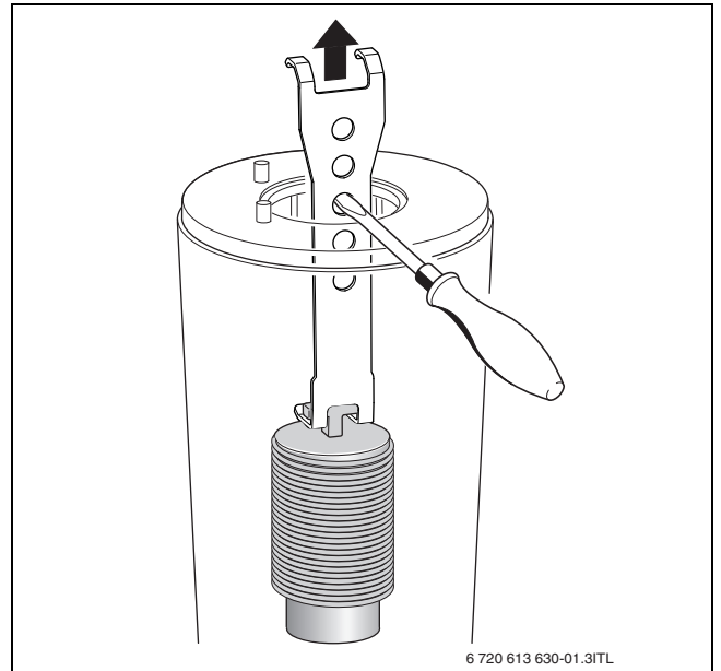
Мал. 63 Виймання нижнього елемента теплообмінника, що служить для оптимізації розподілювання тепла
