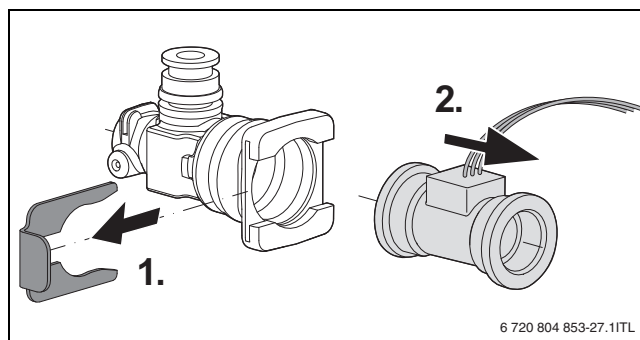
Мал. 71 Демонтаж турбіни на трубі холодної води
