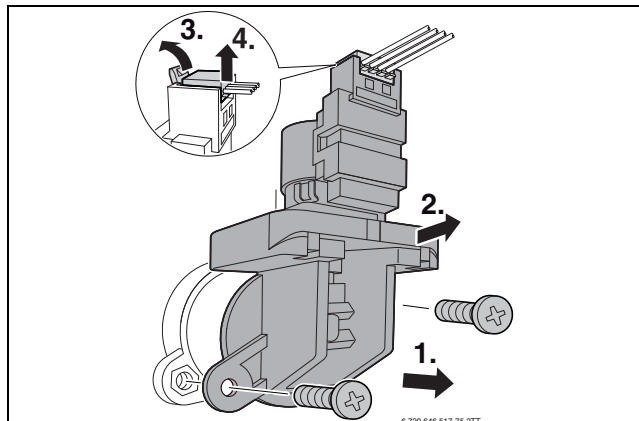
Мал. 74 Зняття 3-ходового клапана
