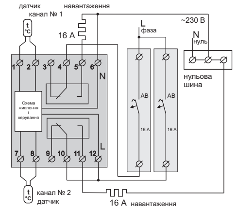
Схема 2. Підключення двох каналів, кожне на окреме навантаження
