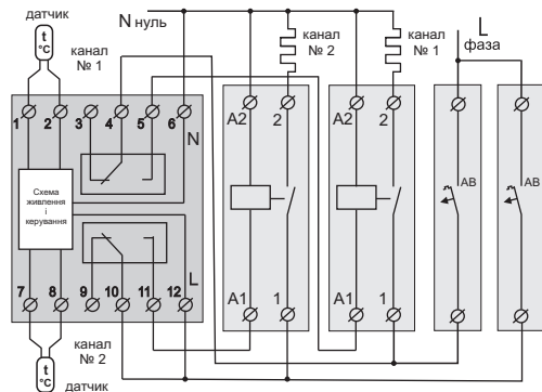
Схема 4. Використання контактора для збільшення комутованої потужності каналу
