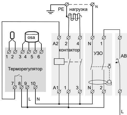
Схема 2. Подключение через контактор
