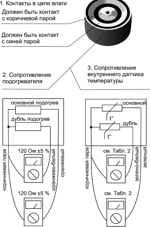
Рисунок 7. Устройство датчика осадков OSA
