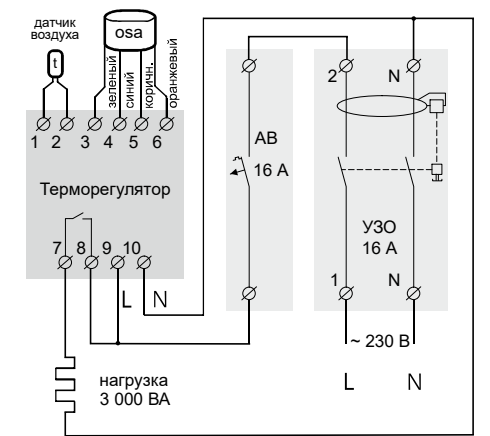
Схема 1. Подключение автоматического выключателя и УЗО
