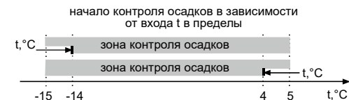
Рисунок 5. Стандартные пределы с гист. 1 °C.
