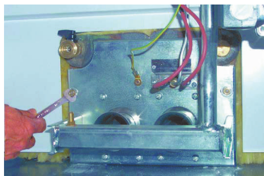
рис. 20 - Демонтаж горелок
