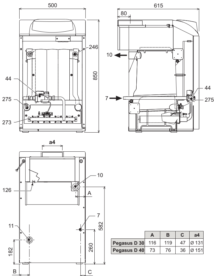
мал. 23 - Розміри, приєднання мод. PEGASUS D 30 E PEGASUS D 40
