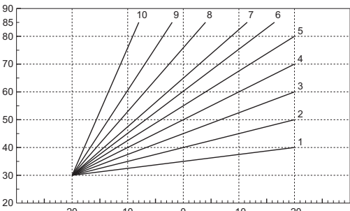
рис. 11 - Компенсационные характеристики
