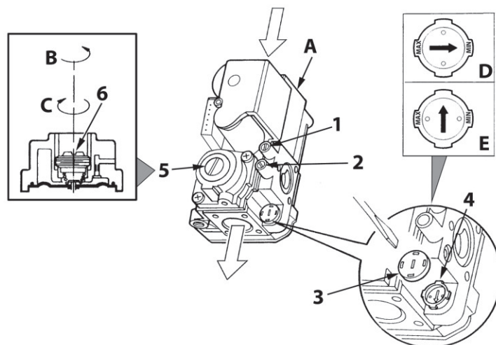
мал. 17 - Регулювання тиску
