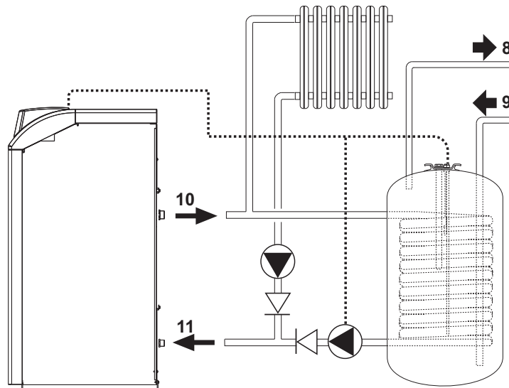
мал. 14 - Схема під'єднання до зовнішнього бойлера
