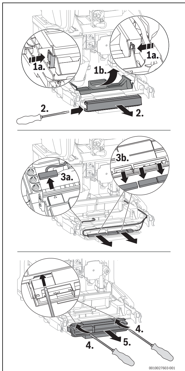
Мал. 140 Витягніть систему керування
