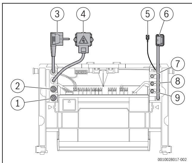
Мал. 76 Стан постачання системи керування з підключеними компонентами
