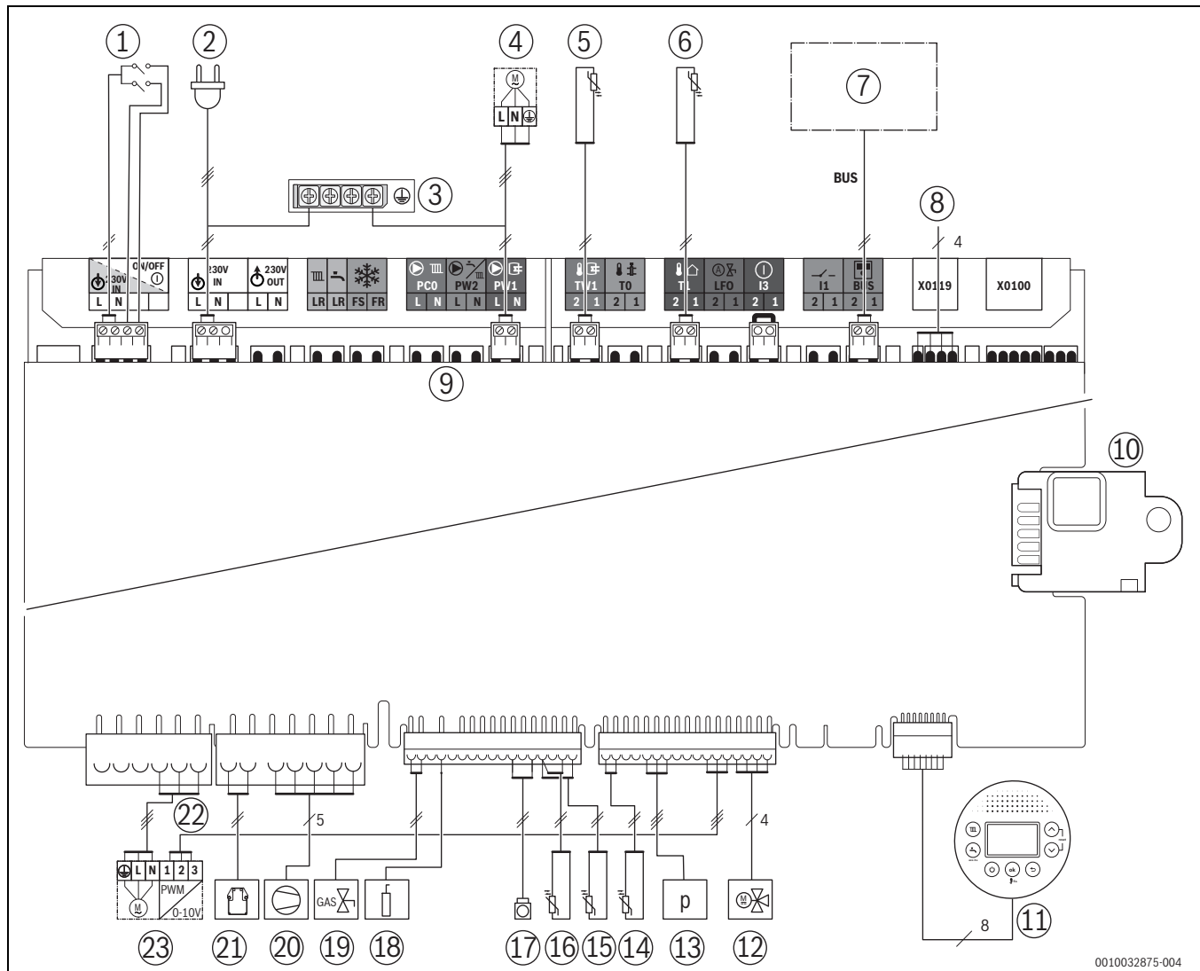
Мал. 149 Електричні підключення
