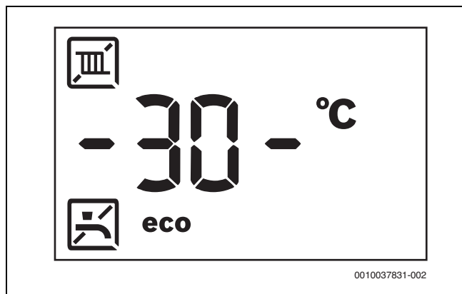
Мал. 96 Температура лінії подачі знаходиться між позначками, що блимають
