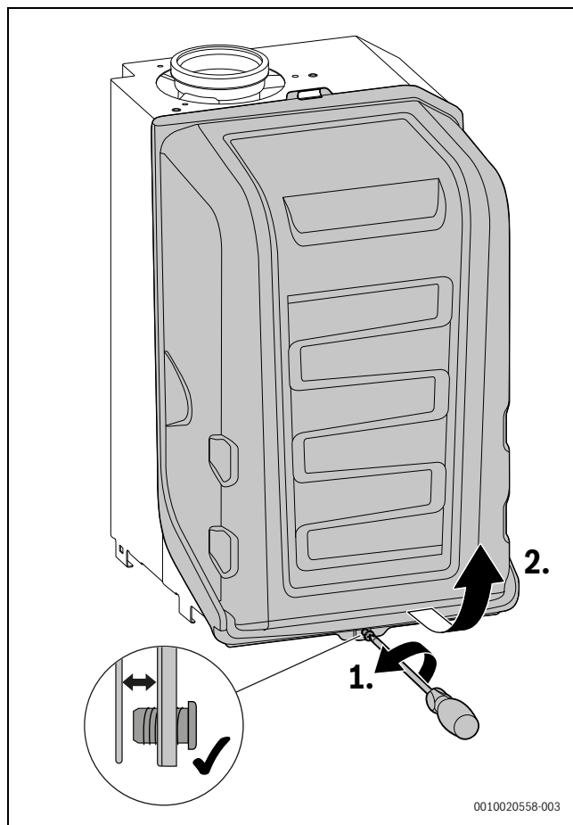
Мал. 107 Зніміть кришку пальника
