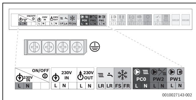
Мал. 79 Діапазон мережевої напруги: клемна колодка
