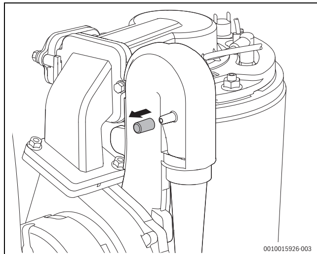
Мал. 109 Штуцер для вимірювання на змішувальній камері
