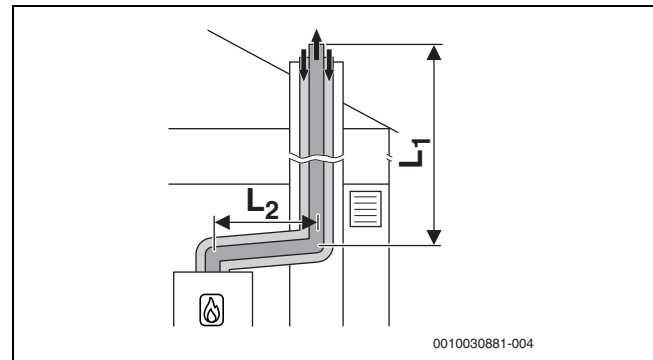
Мал. 23 Концентрична система транспортування повітря для горіння та димових газів згідно з C 33x у шахті
