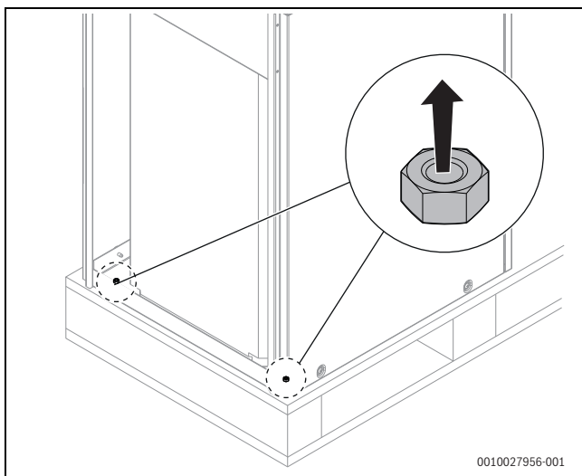
Мал. 43 Зніміть нижній транспортний запобіжник на зворотній стороні бака
