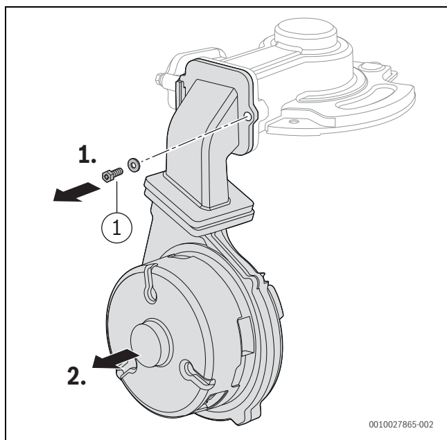
Мал. 115 Демонтаж вентилятора зі змішувальною камерою
