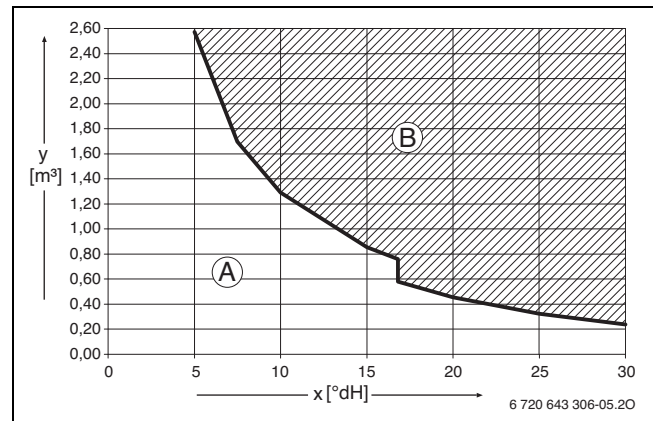
Мал. 37 Вимоги до води для заповнення та підживлення в °dH для приладів потужністю < 50 кВт
