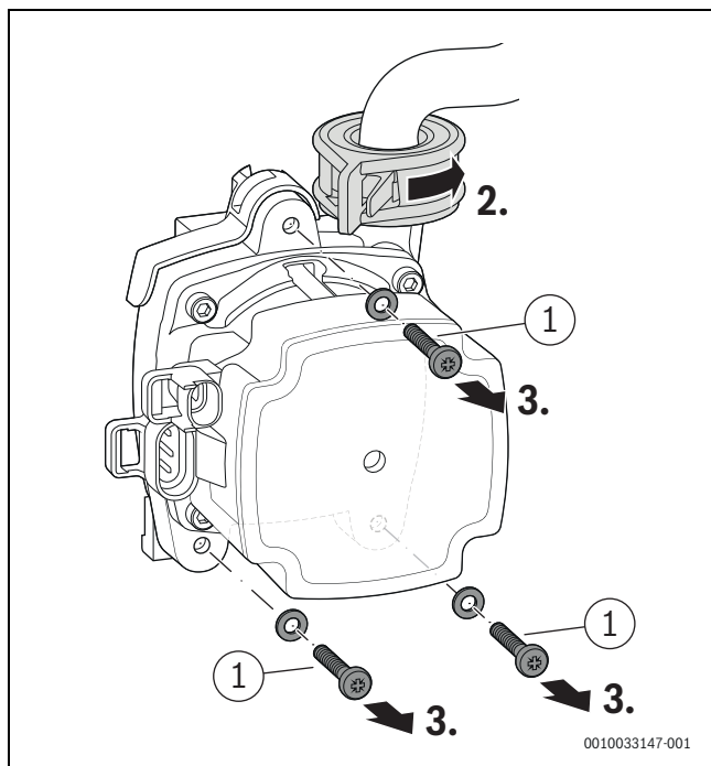
Мал. 129 Розблокуйте насос опалювального контуру та зніміть гвинти
