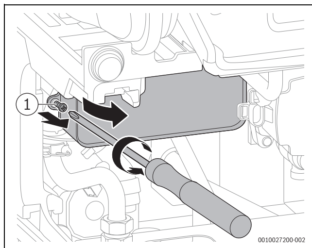
Мал. 145 Демонтаж пластинчастого теплообмінника
