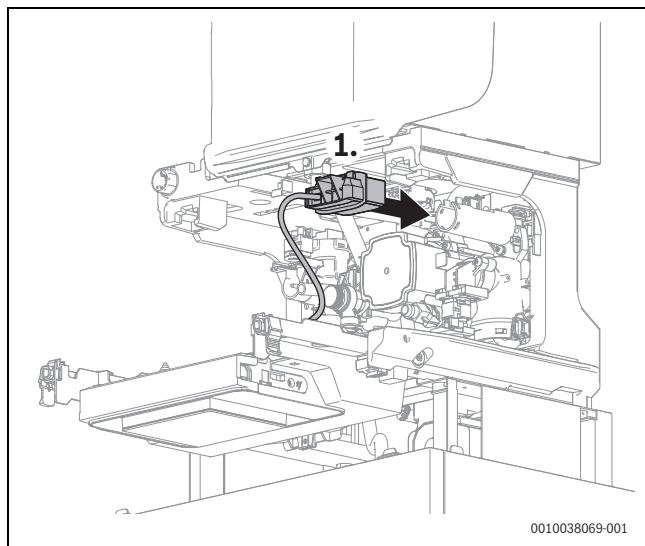
Мал. 58 Спрямуйте тримач Key до задньої частини пристрою
