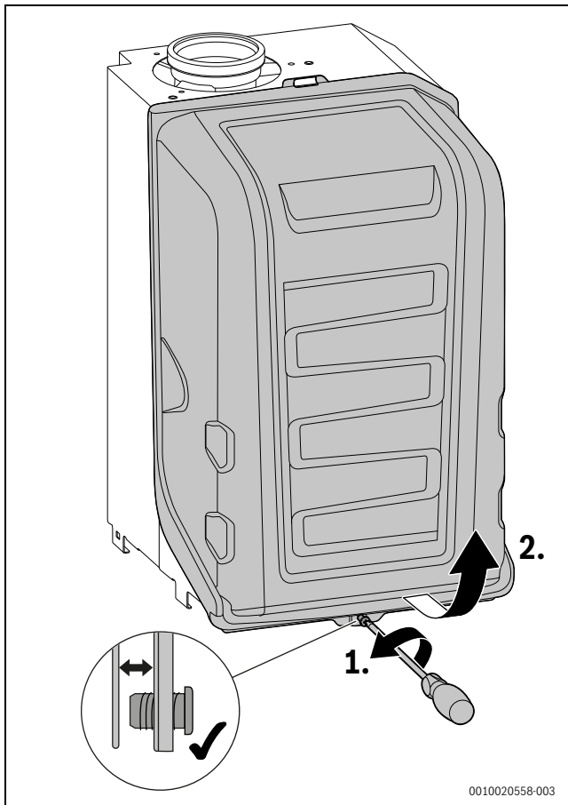
Мал. 70 Зніміть кришку пальника
