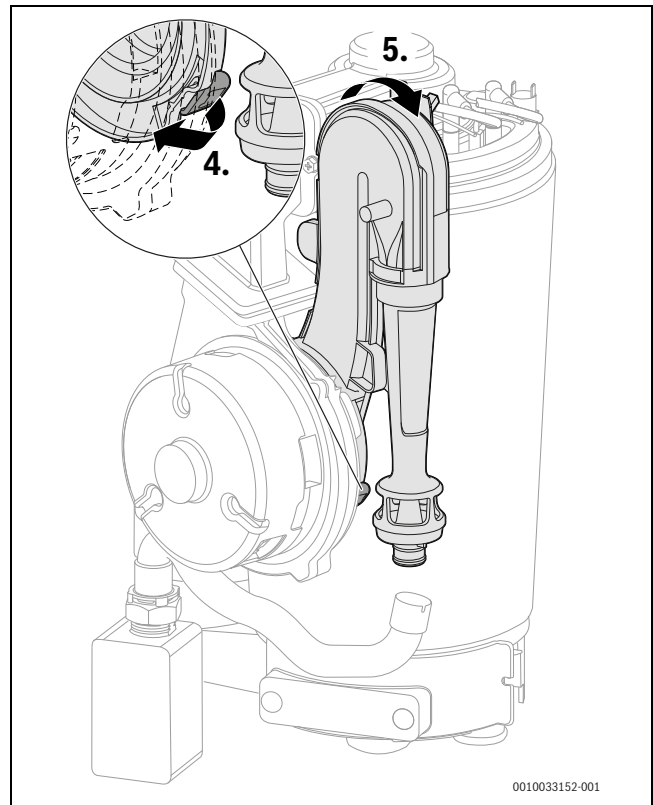
Мал. 112 Знімання трубки Вентурі
