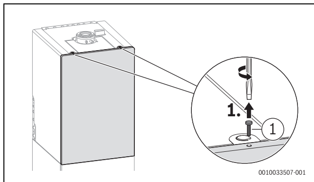
Мал. 105 Відкрутіть запобіжний гвинт
