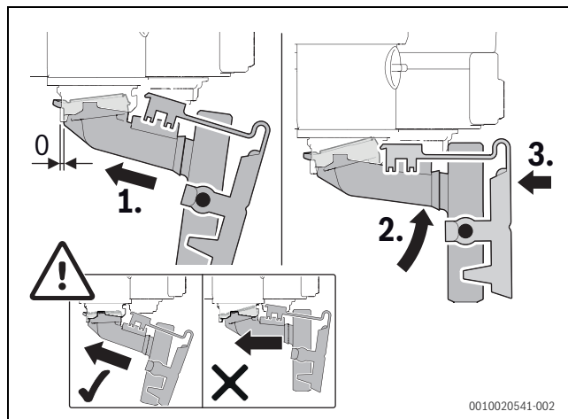
Мал. 144 Встановлення сифону для відведення конденсату
