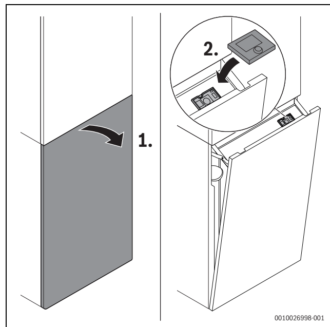
Мал. 68 Вставте блок керування CW 400
