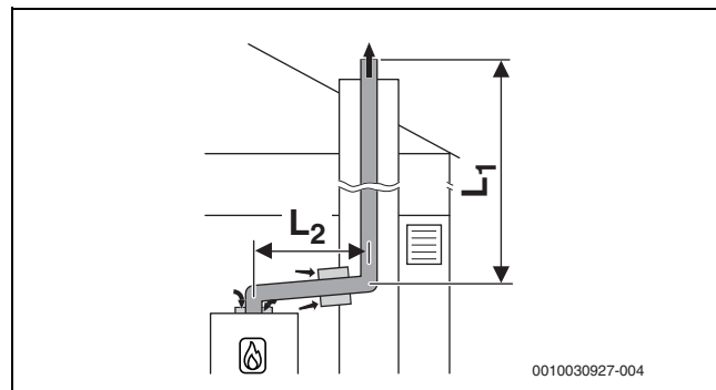
Мал. 30 Система відведення димових газів у шахті жорсткої конструкції відповідно до B_{53p} з подачею повітря у прилад з приміщення та концентричною з'єднувальною деталлю між котельним приміщенням та шахтою
