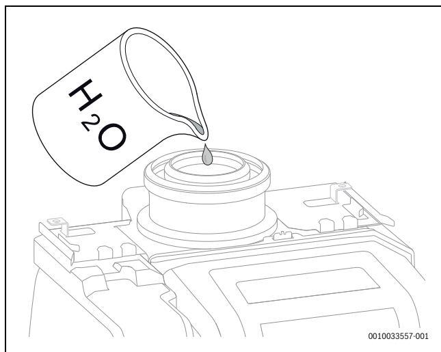
Мал. 65 Наповніть сифон для відведення конденсату водою
