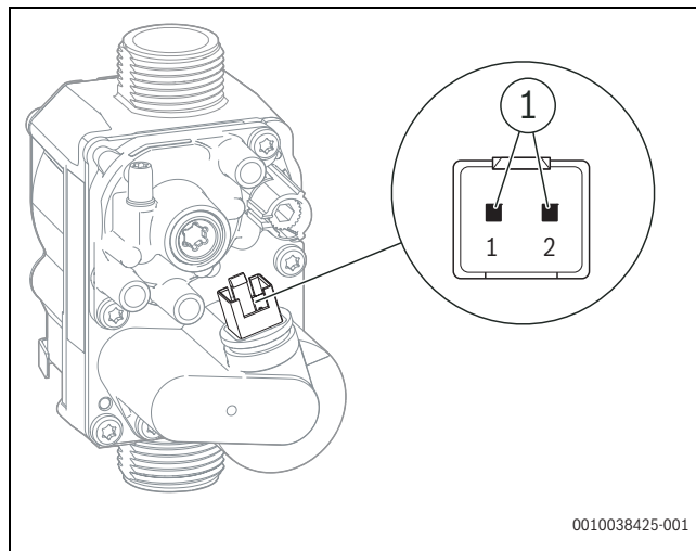
Мал. 110 Точки вимірювання на газовій арматурі
