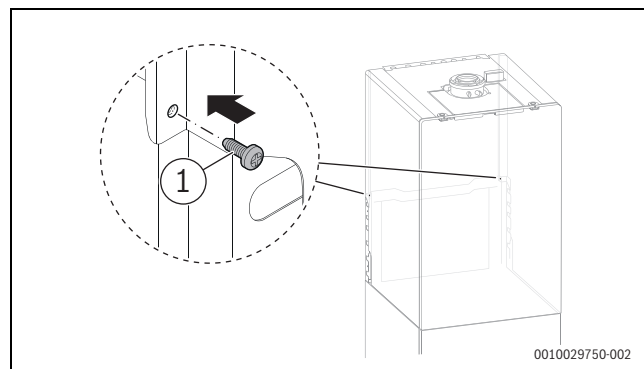
Мал. 88 Затягніть бокові панелі кожуху з лівої та правої сторони
