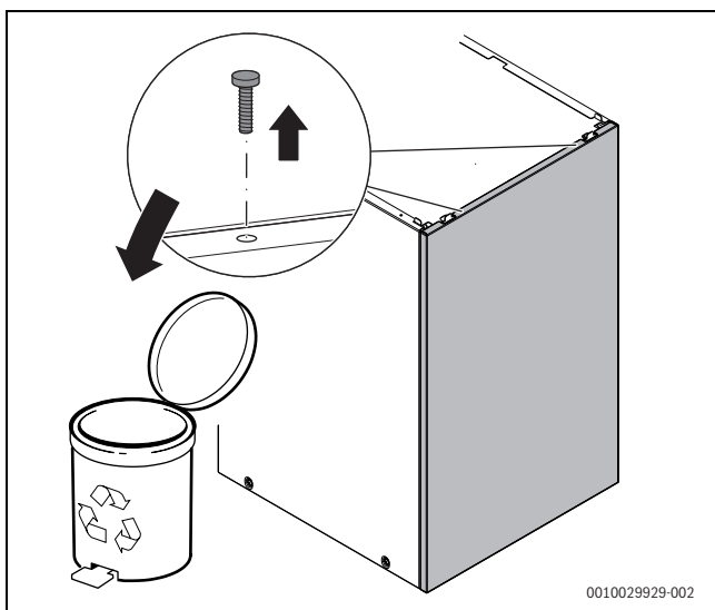
Мал. 44 Зніміть транспортний запобіжник на передній частині кожуха бака
