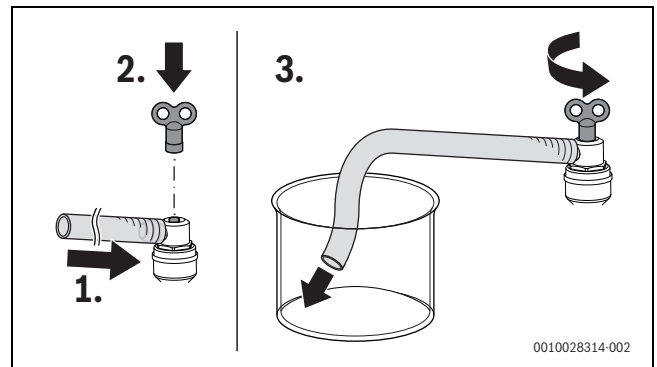
Мал. 71 Видалення повітря з контуру гарячої води та з опалювального контуру
