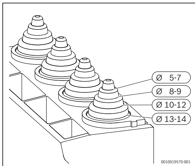
Мал. 78 Підгонка фіксатора проводу до діаметра кабелю
