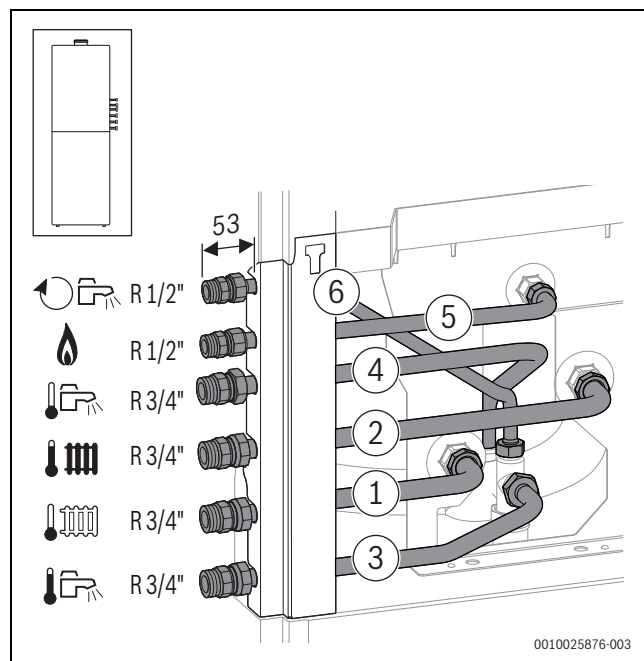
Мал. 46 Додаткові комплектуючі CS 10 з правої сторони змонтовані
