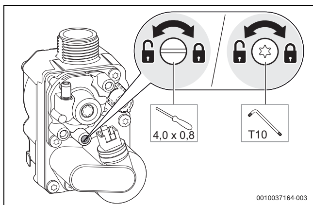
Мал. 98 Вимірювання тиску підключення газу
