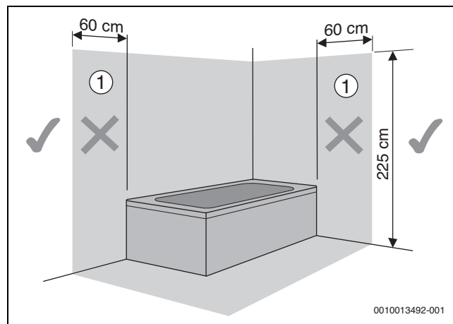
Мал. 36 Захисні зони
