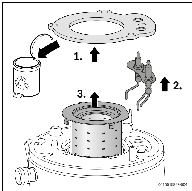
Мал. 117 Виймання пальника
