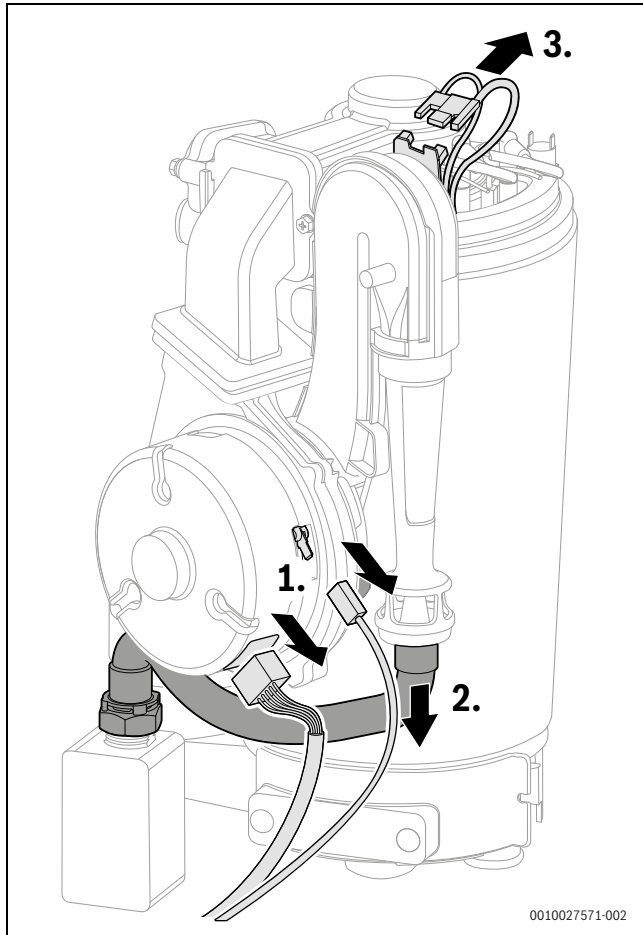
Мал. 111 Зніміть штекер і газовий шланг
