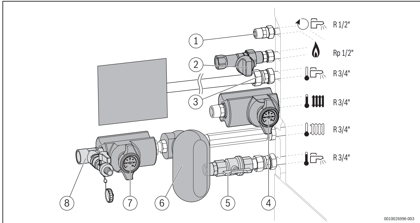
Мал. 69 Додаткові комплектуючі комплекту арматури CS 28-1 – Приклад: горизонтальні з'єднання на лівій стороні
