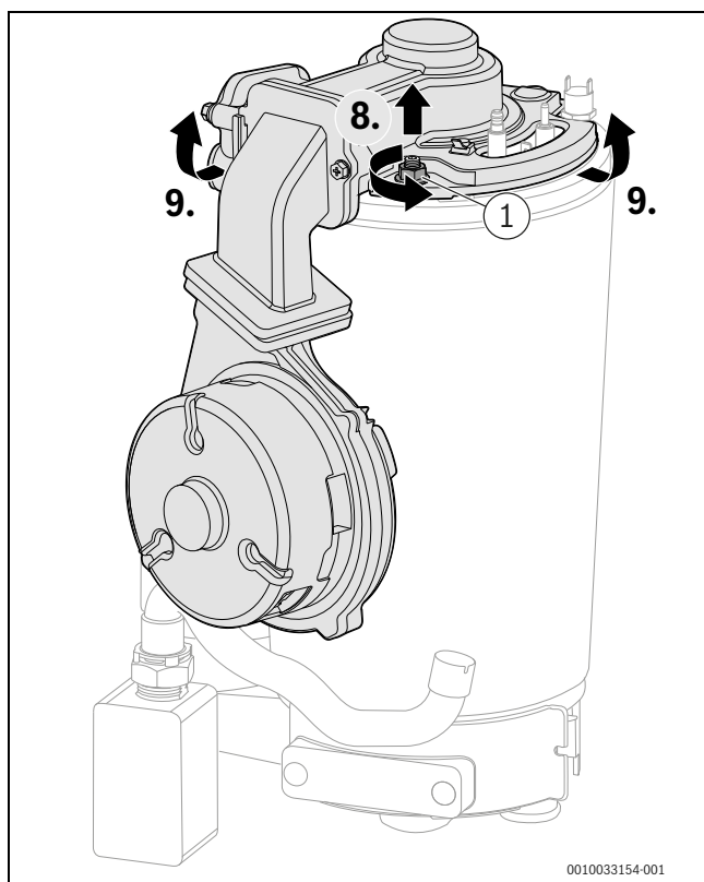
Мал. 114 Знімання кришки пальника разом з вентилятором та змішувальною камерою
