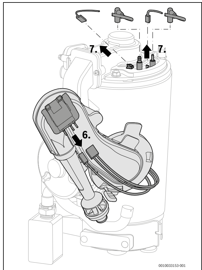
Мал. 113 Знімання кабелів
