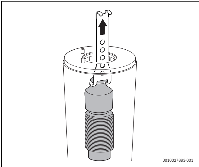
Мал. 118 Виймання верхнього елемента теплообмінника, що служить для оптимізації розподілювання тепла
