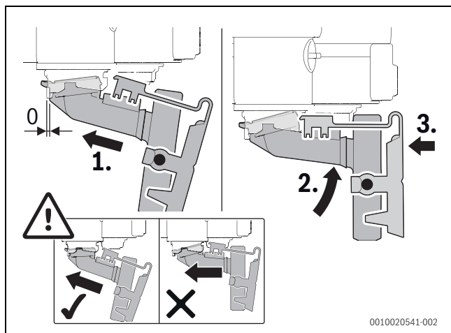
Мал. 57 Вставте назад сифон для відведення конденсату та перевірте надійність його посадки
