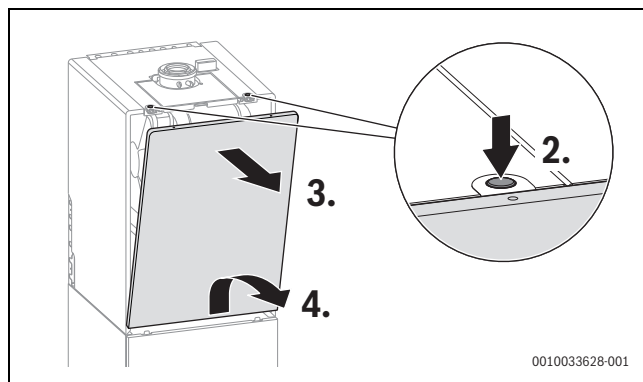
Мал. 106 Знімання передньої частини кожуху
