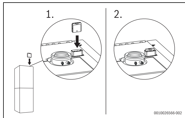
Мал. 67 Встановлення Control Key у тримач Key
