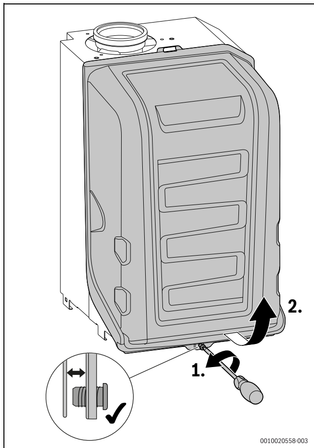
Мал. 97 Зніміть кришку пальника
