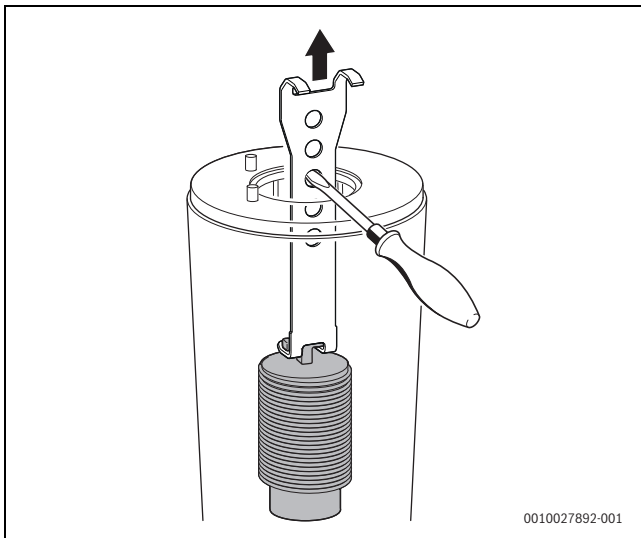
Мал. 119 Виймання нижнього елемента теплообмінника, що служить для оптимізації розподілювання тепла
