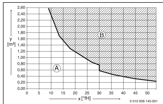
Мал. 38 Вимоги до води для заповнення та підживлення в °fH для приладів потужністю < 50 кВт
