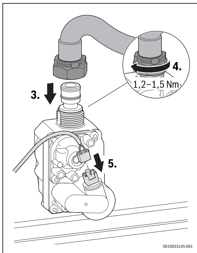
Мал. 139 Притягніть газовий шланг і штекер – Дотримуйтесь моменту затягування
