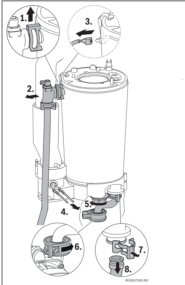
Мал. 126 Від'єднання труби лінії подачі, зняття кабелю та зняття труби зворотної лінії
