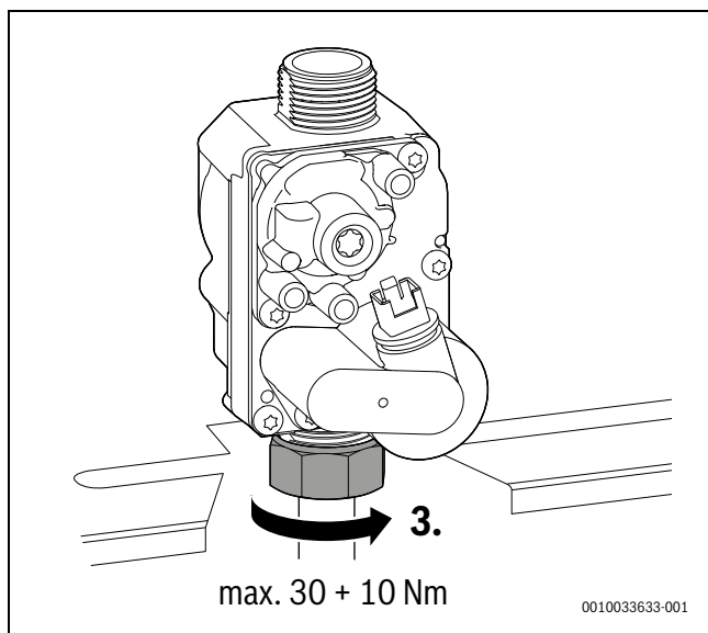
Мал. 137 Дотримуйтесь моменту затягування
