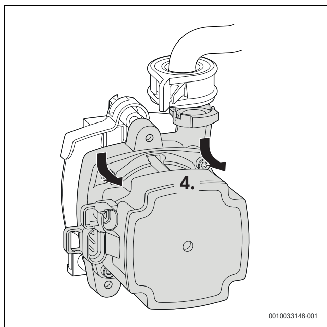
Мал. 130 Знімання насоса опалювального контуру
