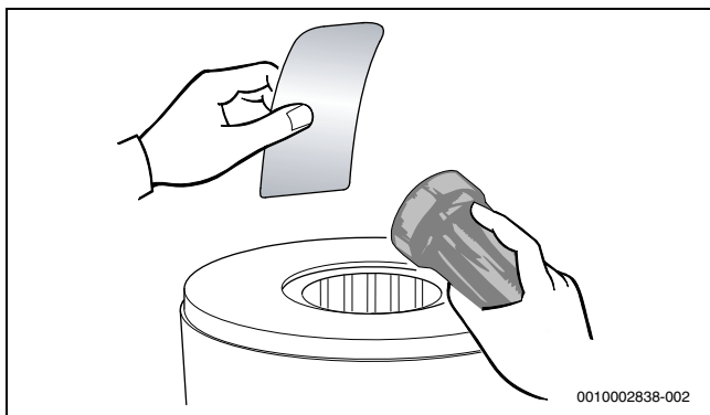
Мал. 124 Перевірка котлового блоку, який включає камеру згорання і теплообмінник, на наявність відкладень
