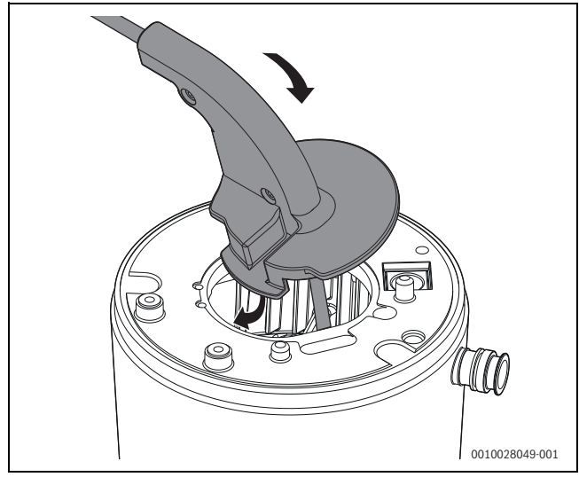
Мал. 120 Вставте щітку у котловий блок, який включає камеру згоряння і теплообмінник
