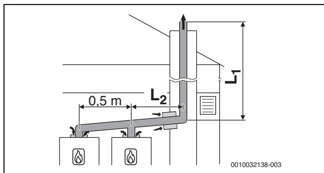
Мал. 34 Каскад з 2 приладами: система відведення димових газів жорсткої конструкції у шахті згідно з В 53p з подачею повітря у прилад з приміщення
