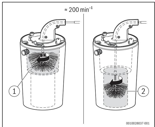
Мал. 122 Чищення котлового блоку, який включає камеру згоряння і теплообмінник (200 об/хв, тільки при правосторонньому обертанні)
