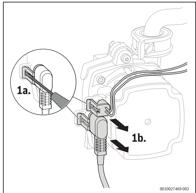
Мал. 128 Зніміть штекер з насоса опалювального контуру
