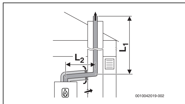
Мал. 31 Система відведення димових газів у шахті із жорсткою конструкцією відповідно до B_{53p} з подачею повітря з приміщення через концентричну систему транспортування повітря для горіння та відпрацьованих газів у котельному приміщенні
