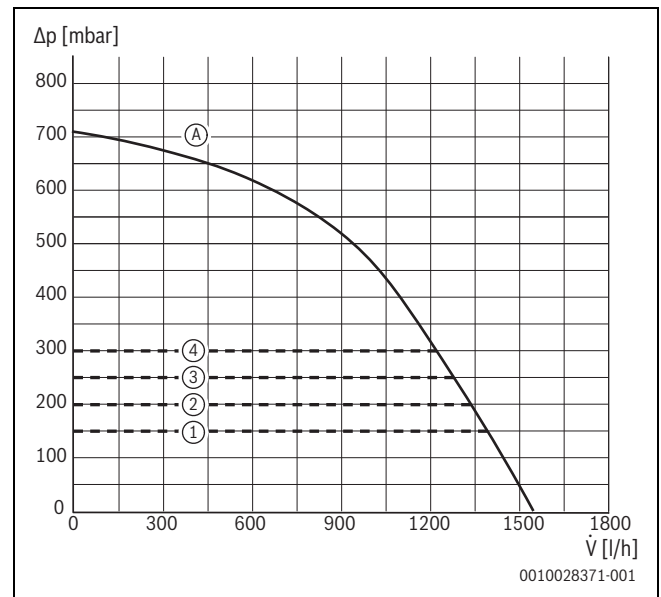
Мал. 150 Характеристики насоса і крива характеристик насоса (17/24 kW)
