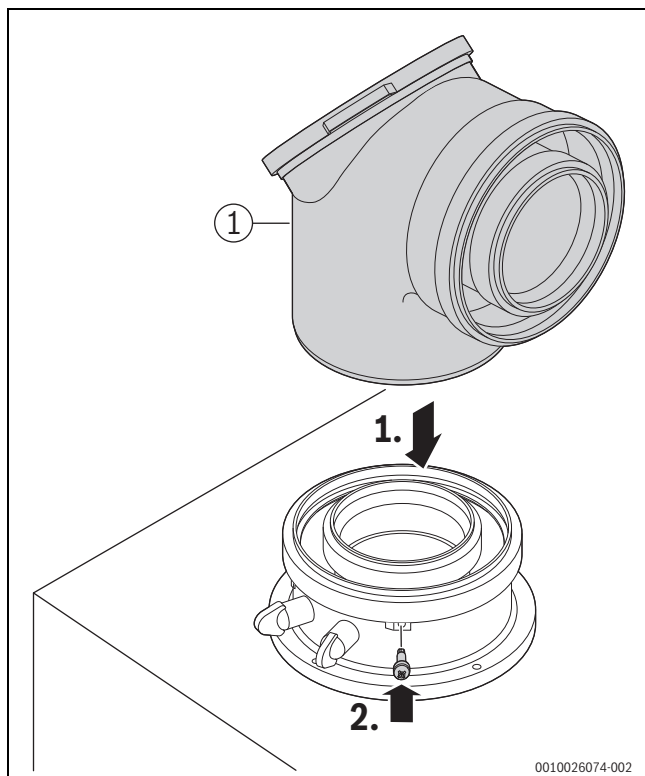
Мал. 66 Встановіть аксесуари для відведення відпрацьованих газів та зафіксуйте гвинтом
