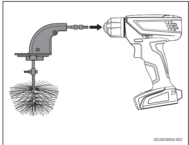
Мал. 121 З'єднайте щітку з акумуляторним шурупвертом
