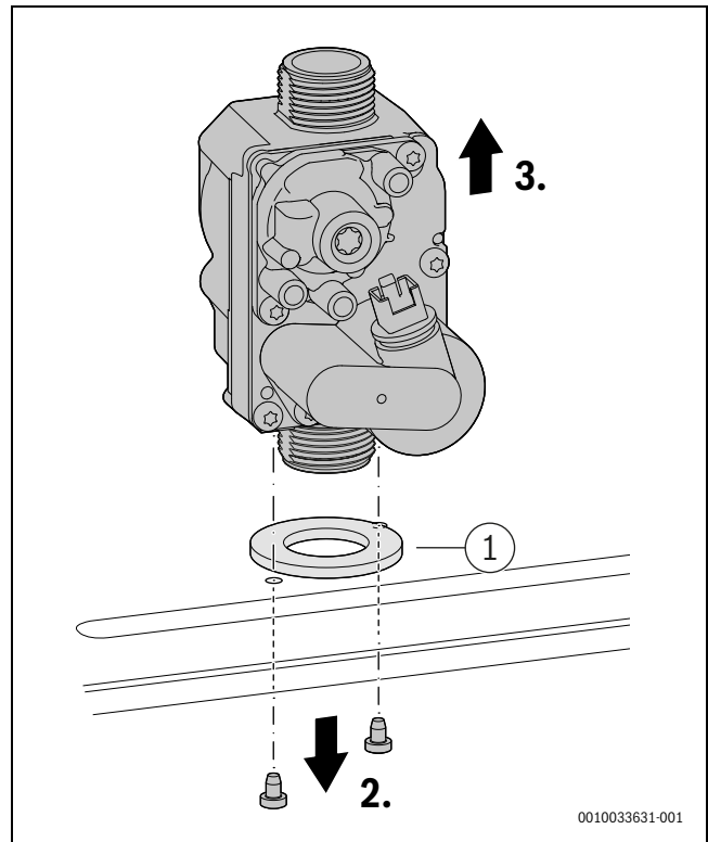
Мал. 135 Демонтаж газової арматури
