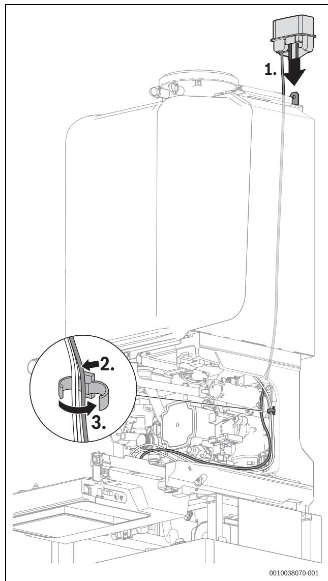
Мал. 59 Вставте тримач Key у роз'єм та зафіксуйте кабель тримачем кабелю
