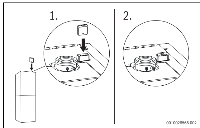
Мал. 2 Встановлення Control Key у тримач Key
