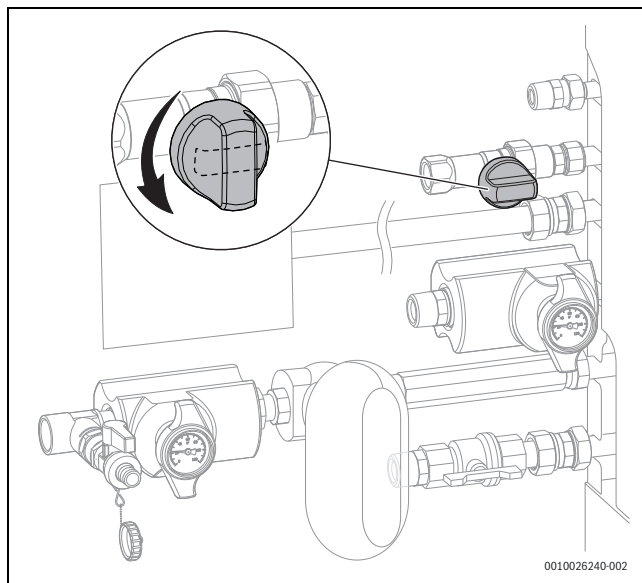
Мал. 5 Відкривання газового крана
