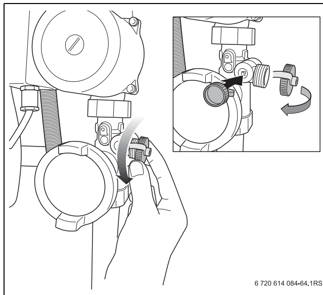
Мал. 3 Запірний ковпачок крану для заповнення та спускання
