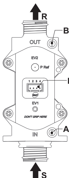
мал. 29 - Газовий вентиль
