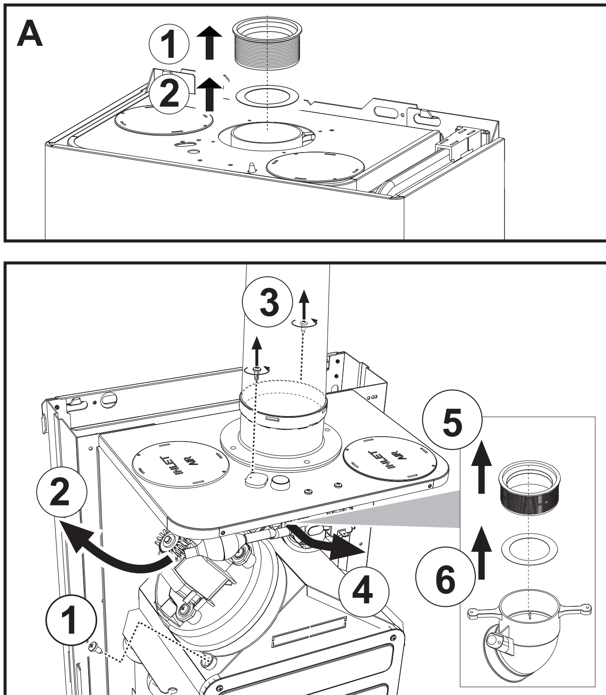
мал. 11- Заміна діафрагми
