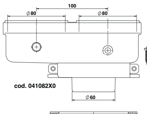
мал. 26- Початковий елемент для відокремлених труб
