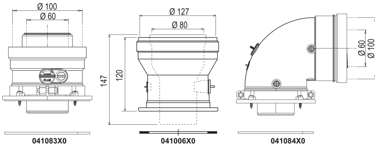
мал. 22- Початкові елементи для коаксіальних трубопроводів
