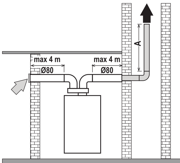
мал. 29- Схема тільки для гнучкої труби
