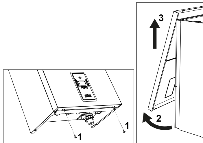
мал. 47- Відкриття передньої панелі
