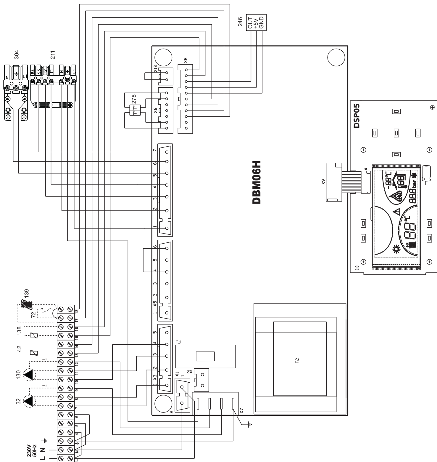
fig. 23 - Schéma électrique
