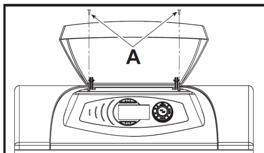
rysunek 17 - Dostęp do elektrycznej skrzynki zaciskowej
