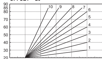
fig. 14 - Voorbeeld van parallele verplaatsing van de compensatiecurven
