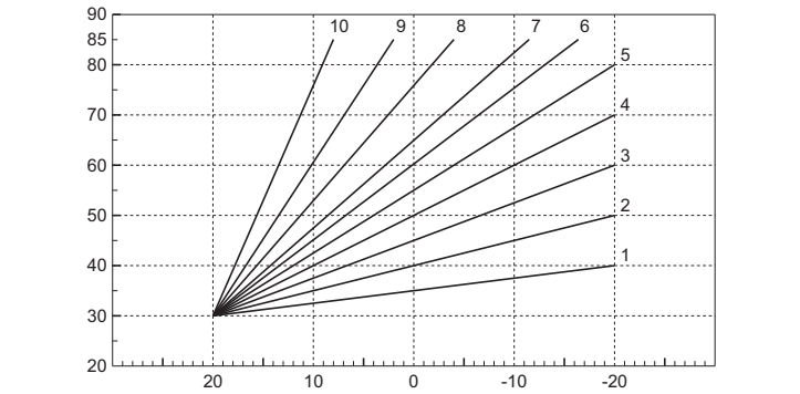
fig. 13 - Curve di compensazione
