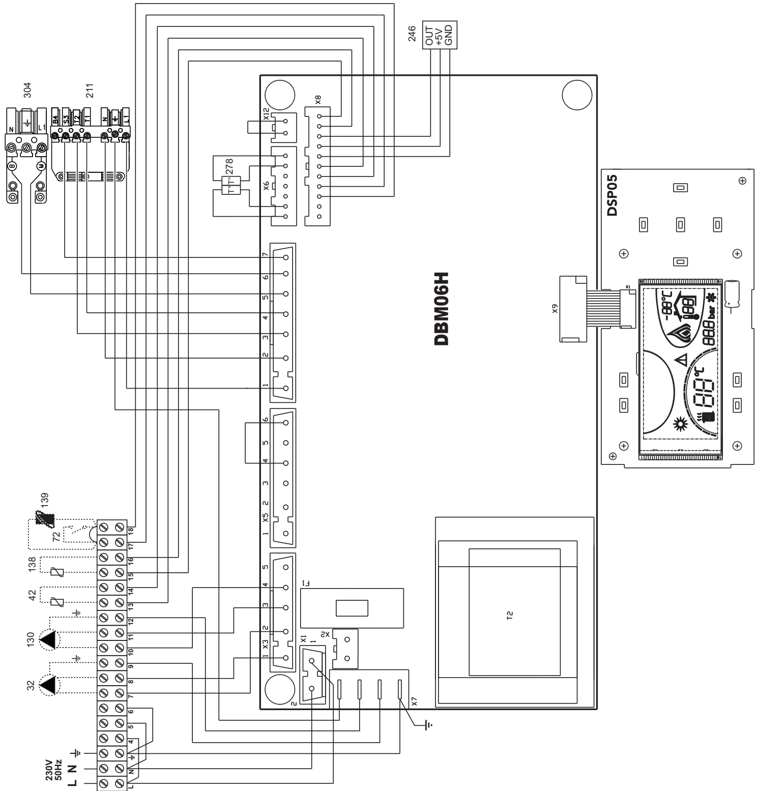
fig. 23 - Wiring diagram
