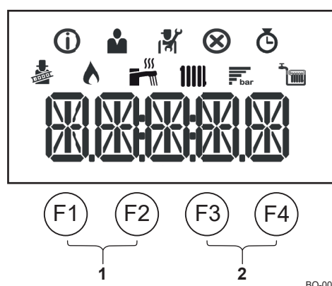
Рис. 8 Опис кнопок
