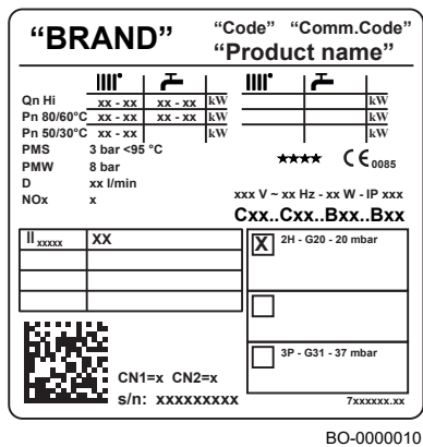
Рис. 12 Ідентифікаційна табличка
