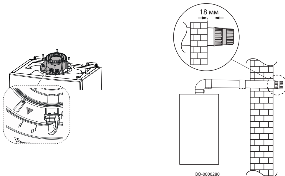
Рис. 23 Коаксіальний димохід
