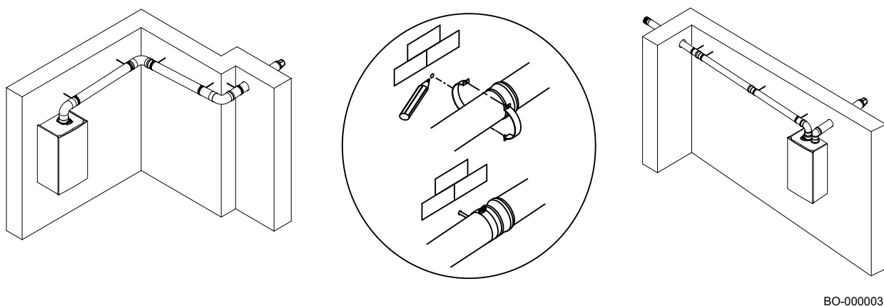
Рис. 21 Спосіб кріплення димохідних патрубків до стіни
