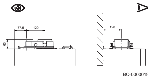
Рис. 26 Роздільні патрубки подачі повітря/видалення димових газів
