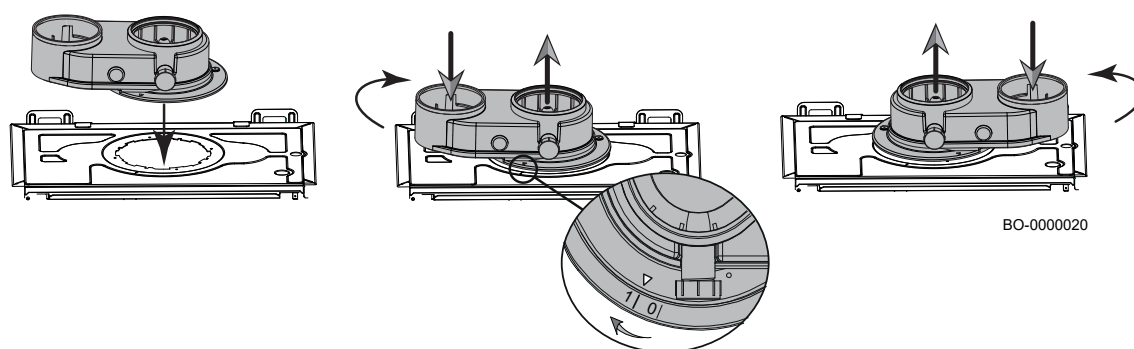
Рис. 27 Монтаж адаптера роздільного дымоходу
