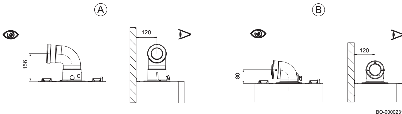
Рис. 22 Адаптер коаксіального димоходу
