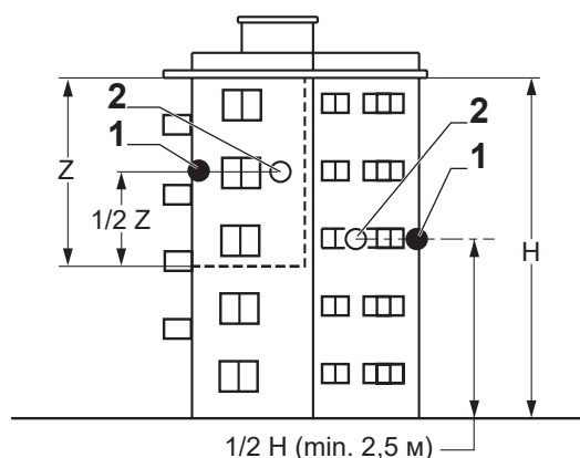
Рис. 17 Рекомендовані місця А
