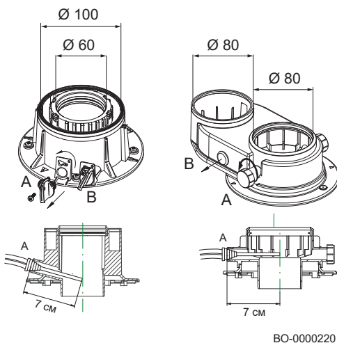
Рис. 41 Тип адаптера димоходу – точка вимірювання димових газів
