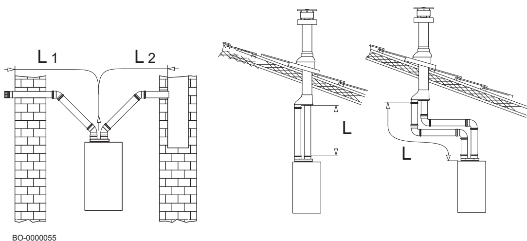
Рис. 28 Приклади монтажу з використанням роздільних дымоходів
