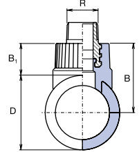
Вварное седло
