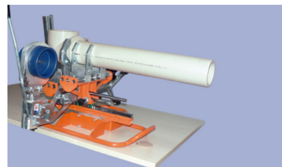
готовое сварное соединение после охлаждения
