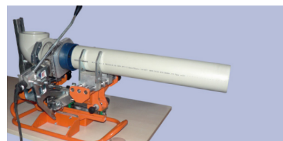
закрепление в аппарате и центровка, потом нагрев
