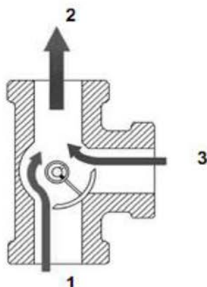
Рис. 6. Триходових змішувальний клапан
