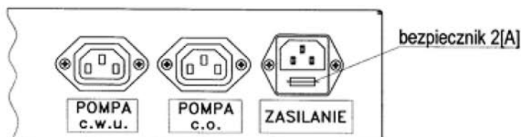
Рис. 10. Приєднання на верхній кришці обудови котла: живлення 230 V 50 Hz, насос с.о., насос с.w.u.
