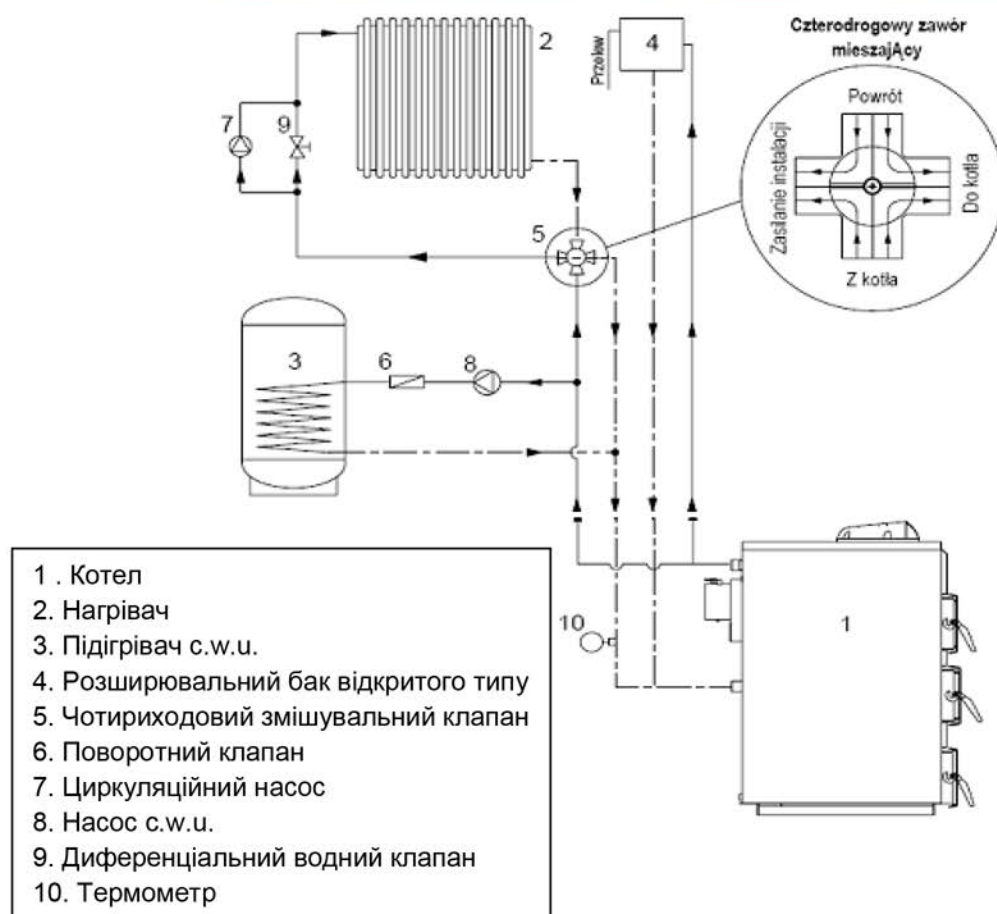
Рис. 7. Схема приєднання котла до опалювальної системи с.о. і с.в.и. з використанням чотириходового змішувального клапана
