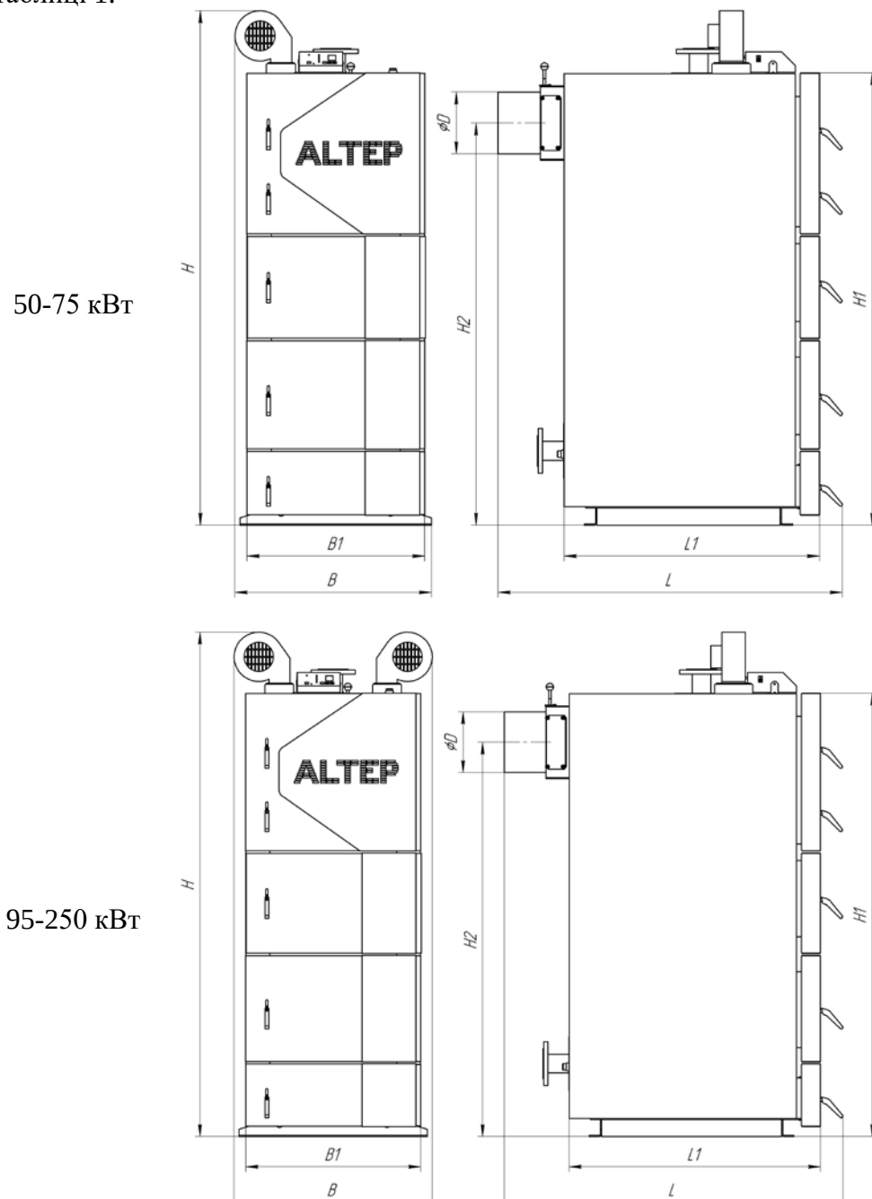
Рисунок 1 – Габаритне креслення котла типу КТ-2Е-N
