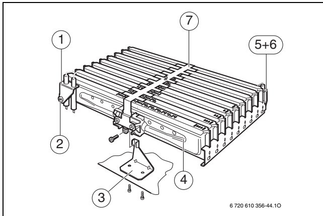
Рис. 31 Модуль пальника
