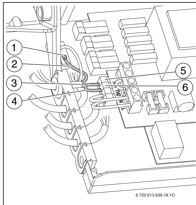
Рис. 15 Підключення мережевого кабелю 230 В ЗС
