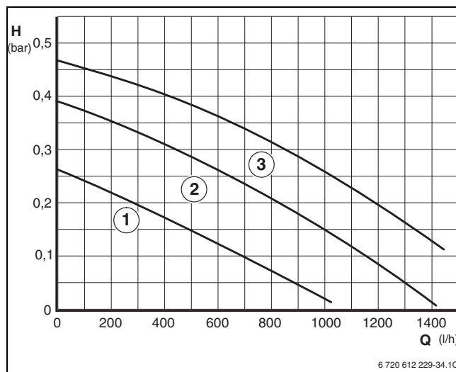
Рис. 25 Графічне зображення характеристик помпи
