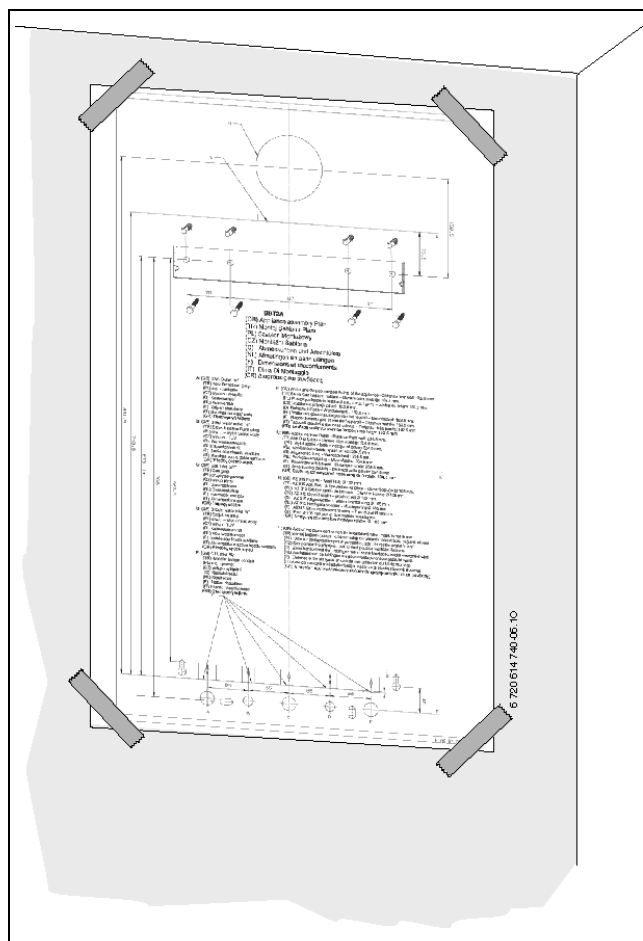
Рис. 7 монтажний шаблон
