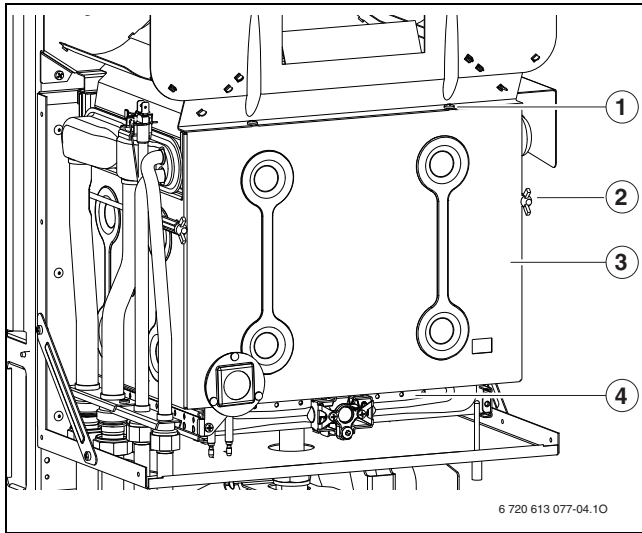
Рис. 30 Відкритий пальник
