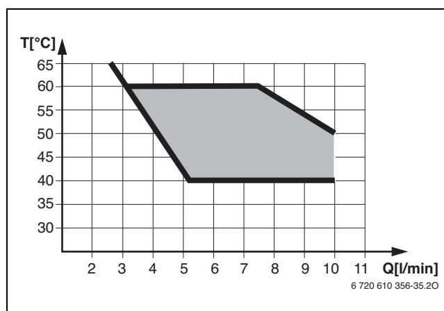
Рис. 20 Діаграма для температури холодної води на вході +15 °C
