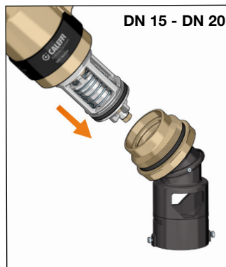
Прикладная схема код 580104/580150
