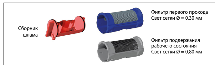
Комплект аксессуара для заполнения и промывки контура и фильтры аксессуары для устройства серии 5453.
